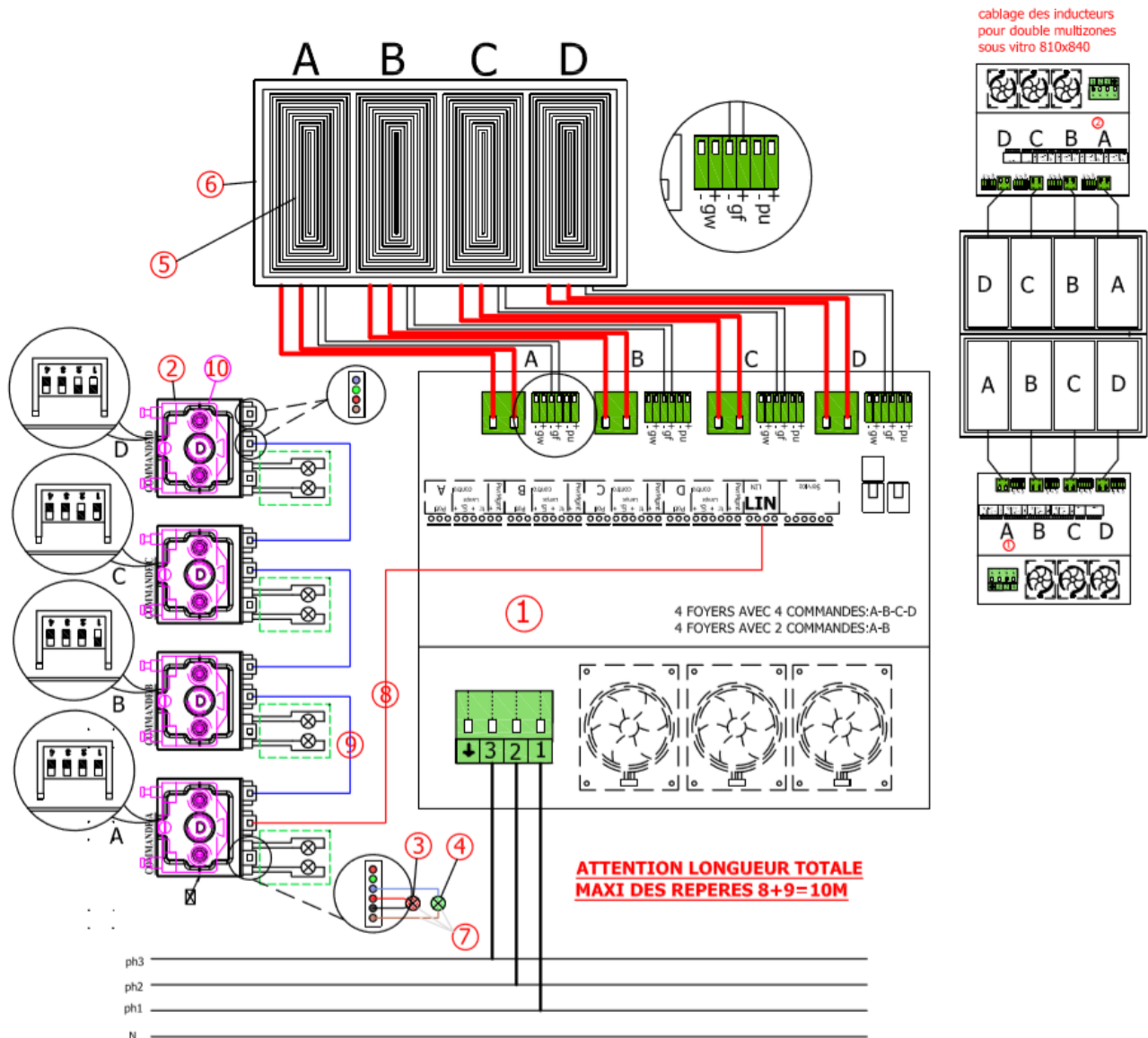
Fig. 2 Schéma électrique induction multizones
